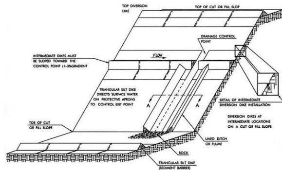
Diversion Dike
